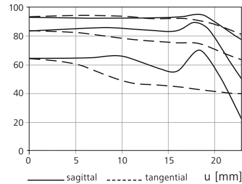
MTF [%], Blendenzahl: k = 4,0
