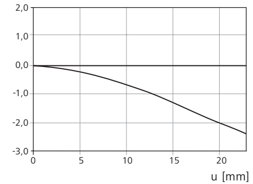
V [%], Verzeichnung
