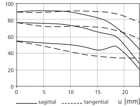
MTF [%], Blendenzahl: k = 2,0
